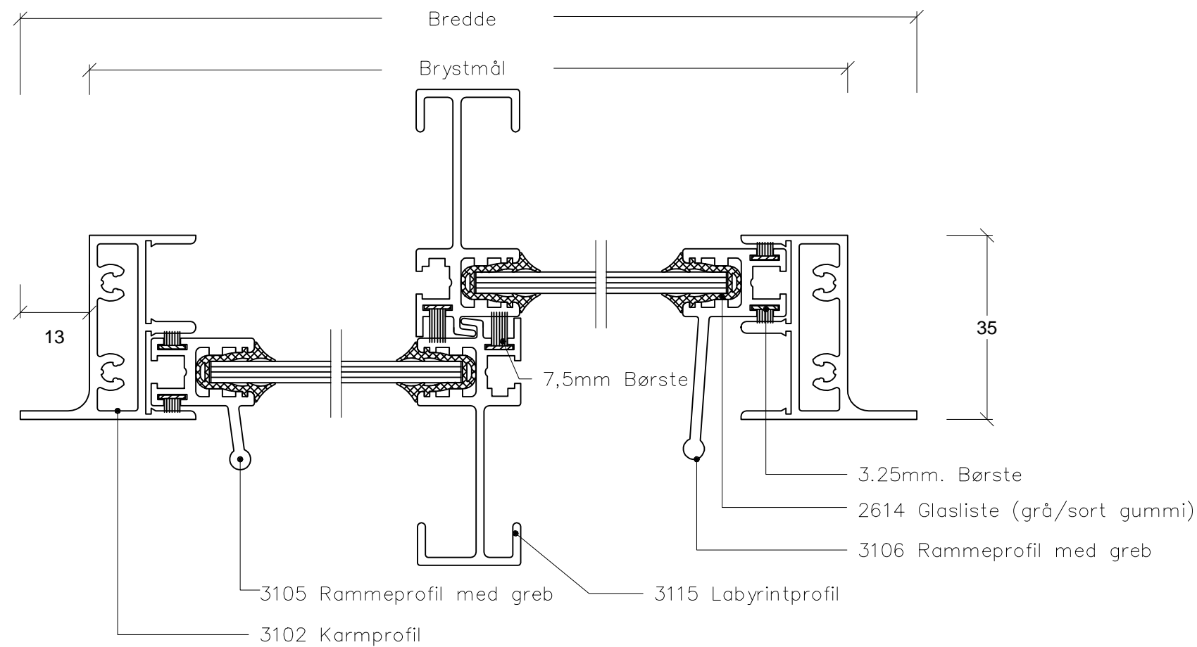
VANDRET SNIT 1:1
