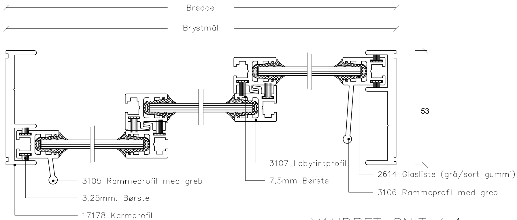
VANDRET SNIT 1:1
