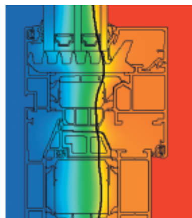
Isothermforløp profilsnitt Schüco vindu AWS 75.SI
