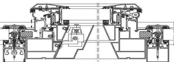
Schüco AWS 57 RO, høy karmprofil, M = 1:8
