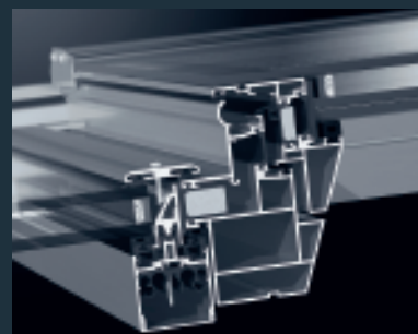
Schüco takluke AWS 57 RO
