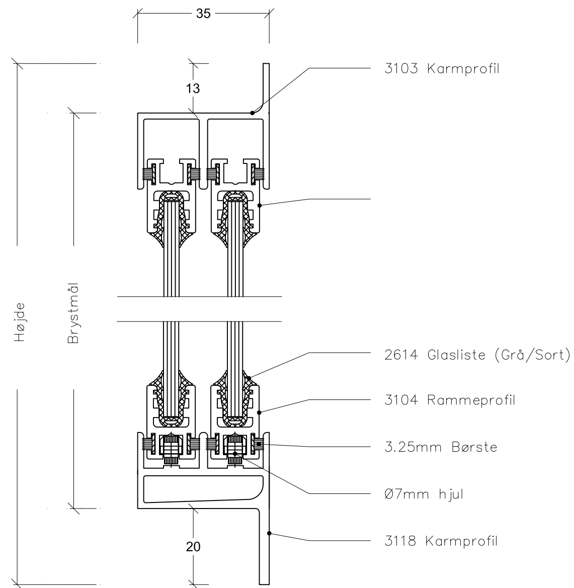
LODRET SNIT 1:1
