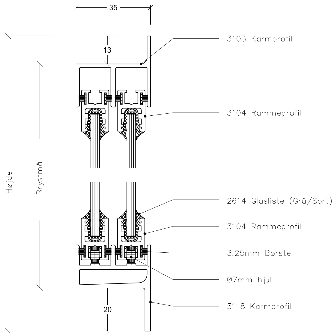
LODRET SNIT 1:1
